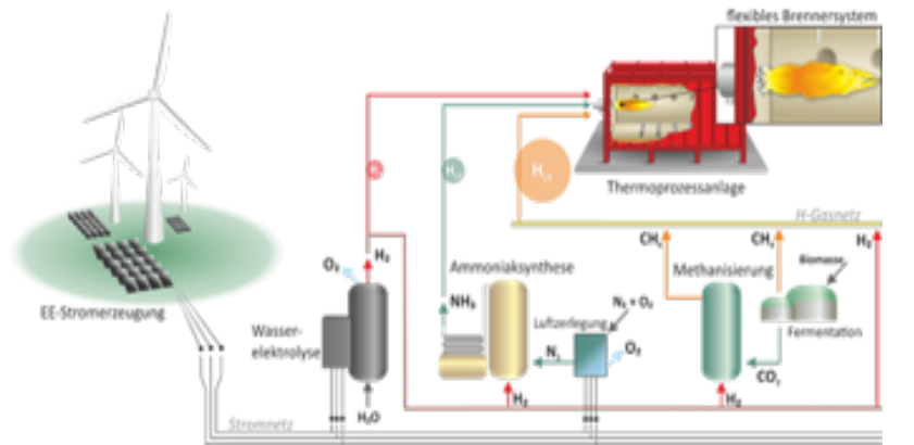
SCHEMATISCHE DARSTELLUNG DER SEMI-INDUSTRIELLEN VERSUCHSINFRASTRUKTUR IM GWI
