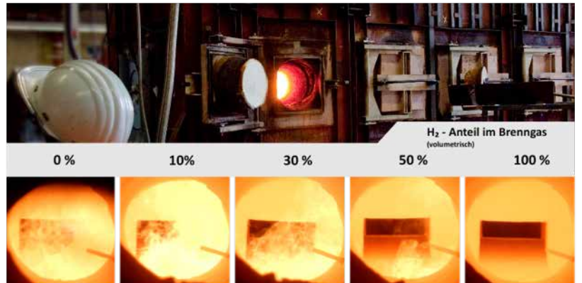
VERSUCHSREIHE ZUR H 2 -BEIMISCHUNG AN DER SEMI-INDUSTRIELLEN ANLAGE
