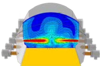
CFD-SIMULATION: STRÖMUNGSFELD EINER GLASSCHMELZWANNE
