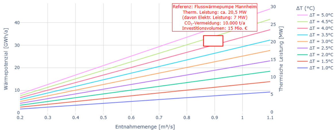
Abbildung 58: Wärmepotenzial und Wärmeleistung in Abhängigkeit der Entnahmemenge bei verschiedenen Temperaturdifferenzen des Entnahmewassers (eigene Darstellung)
