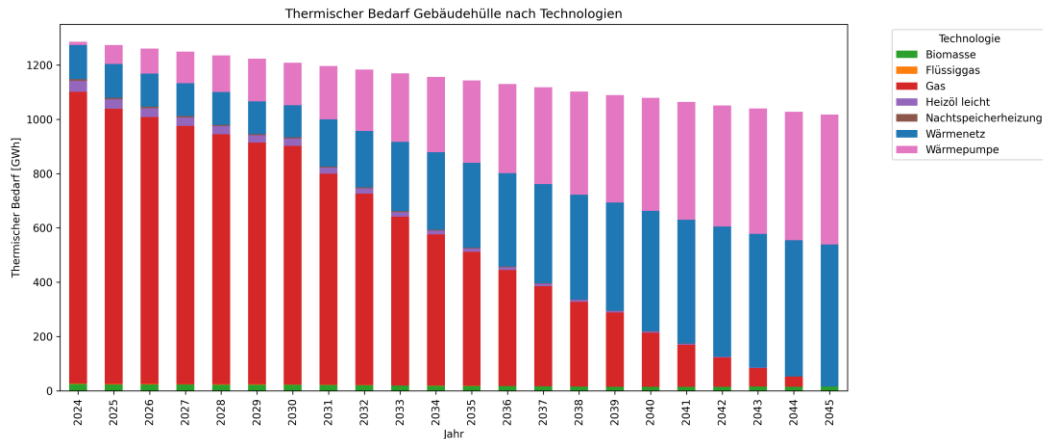
Abbildung 72: Jährliche Entwicklung des Wärmebedarfs der Gebäude nach Technologien im maßgeblichen Zielszenario (eigene Darstellung)
