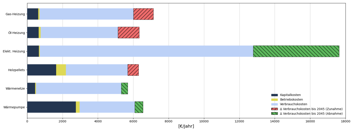
Abbildung 88: Mehrfamilienhaus unsaniert. Wohnfläche = 300m 2 , Wärmeleistung = 20,5 kW, Wärmebedarf = 37 MWh/a (eigene Darstellung)
