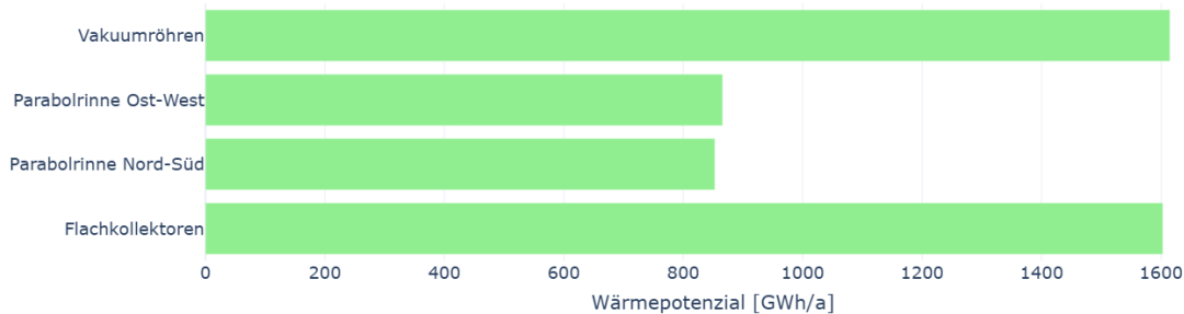
Abbildung 54: Potenzieller jährlicher Freiflächen-Solarthermie Wärmeertrag in GWh/a für unterschiedliche Technologieoptionen (Quelle: LANUK-DFST)
