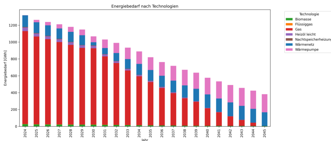
Abbildung 78: Jährliche Entwicklung des Endenergiebedarfs der Gebäude nach Technologien im maßgeblichen Zielszenario (eigene Darstellung)
