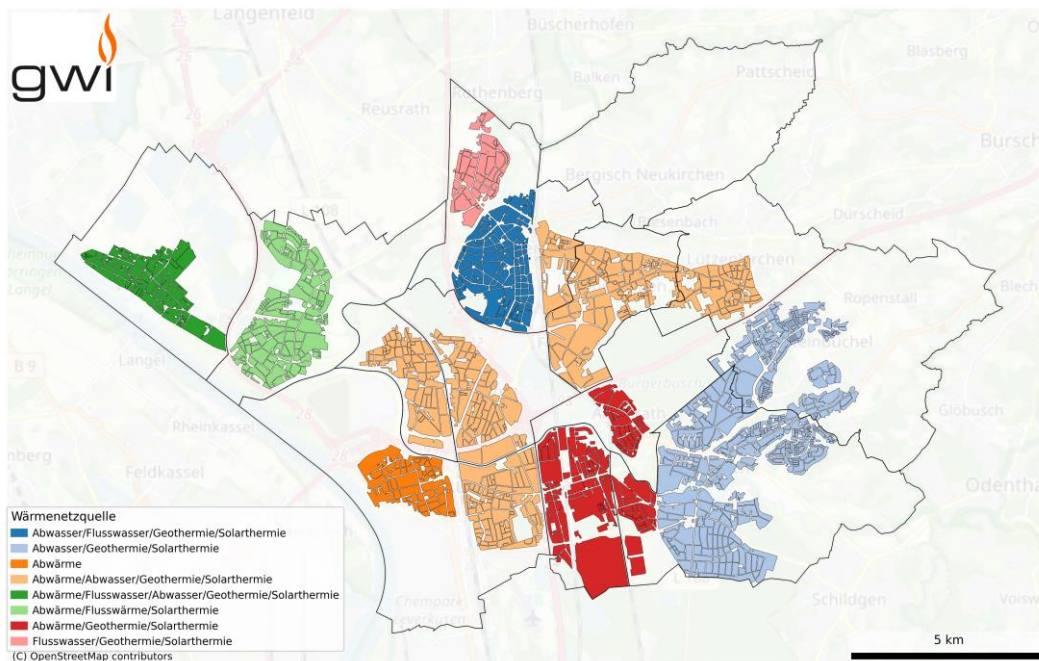
Abbildung 92: Erneuerbare Energiequellen für Wärmenetze (Quelle: ALKIS , LANUK-BB )
