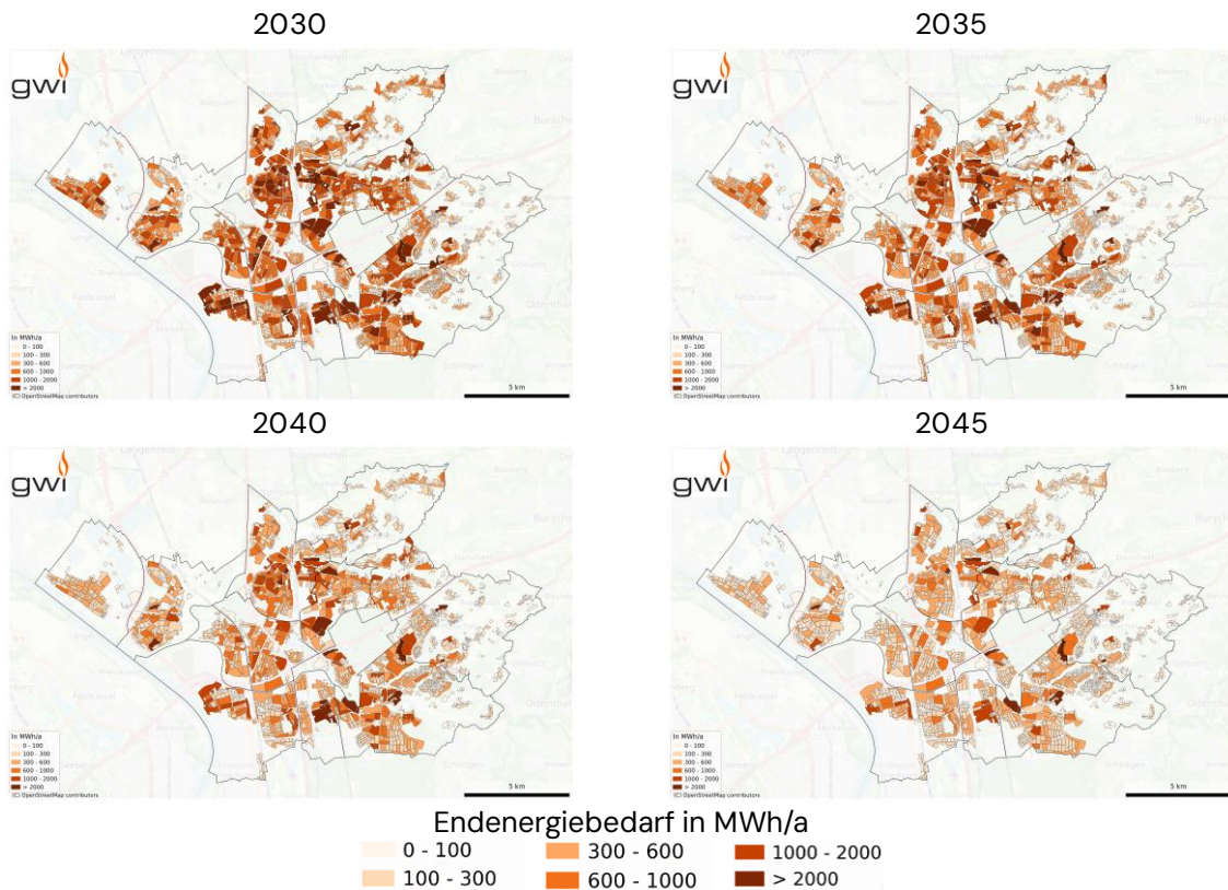
Abbildung 79: Endenergiebedarf im maßgeblichen Zielszenario. Baublöcke mit ausschließlich industrieller Nutzung wurden nicht berücksichtigt (Quelle: ALKIS , LANUK-BB )
