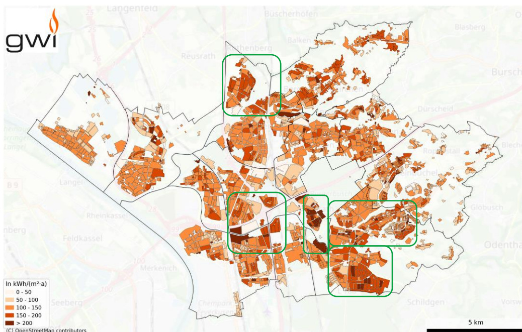
Abbildung 71: Spezifische Wärmebedarfe auf Baublockebene und Gebiete mit erhöhtem Einsparpotenzial. Baublöcke mit ausschließlich industrieller Nutzung wurden nicht berücksichtigt (Quelle: ALKIS , LANUK-BB ).
