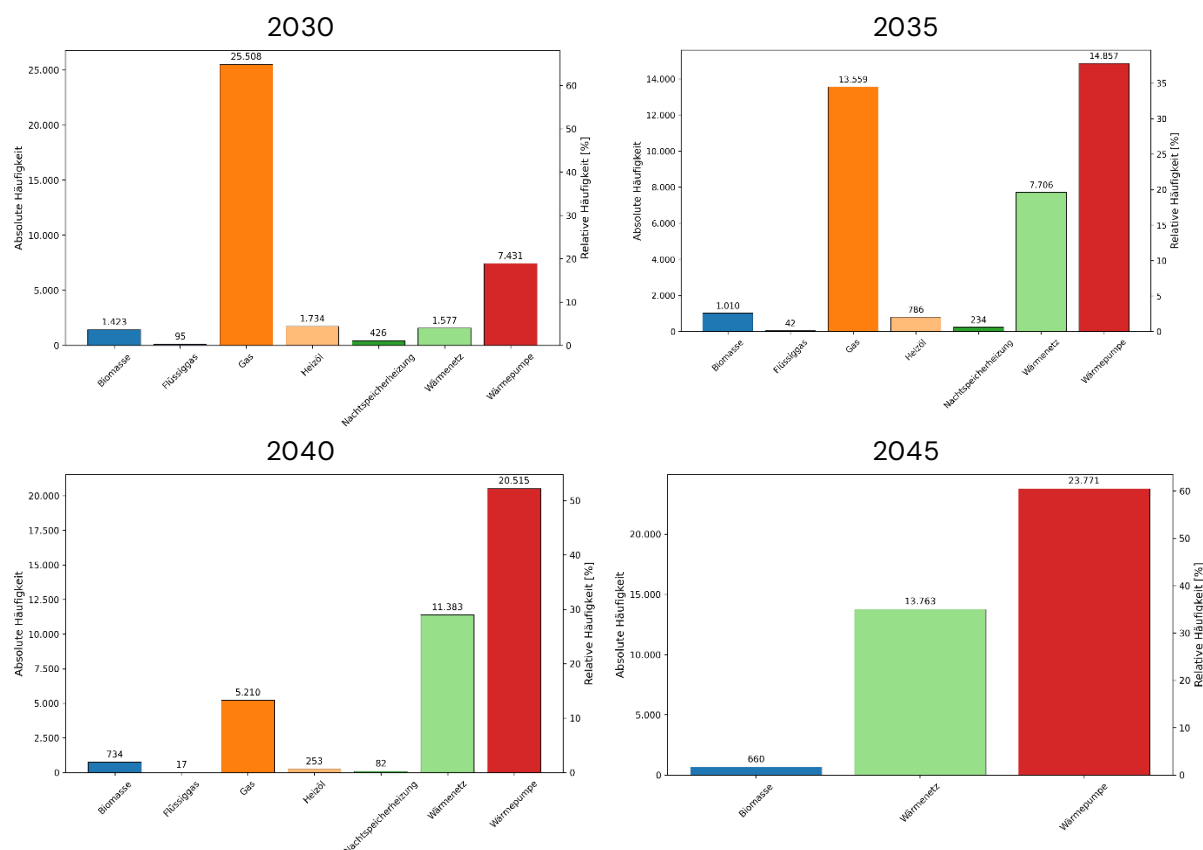
Abbildung 66: Häufigkeit der Technologien auf Gebäudeebene im maßgeblichen Zielszenario. Baublöcke mit ausschließlich industrieller Nutzung wurden nicht berücksichtigt (eigene Darstellung)
