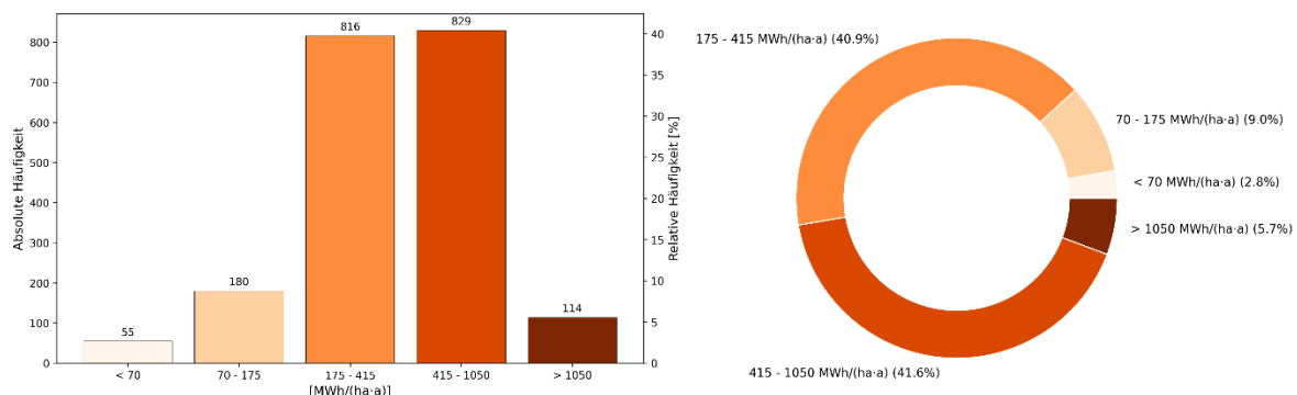
Abbildung 24: Wärmebedarfsdichten der Baublöcke und statistische Verteilung der Bedarfsklassen (Quellen: ALKIS , LANUK-BB , LANUK-RBM , RNG-RLM , RNG-EFH/MFH , RNG-NSH/WP , EVL-FW )
