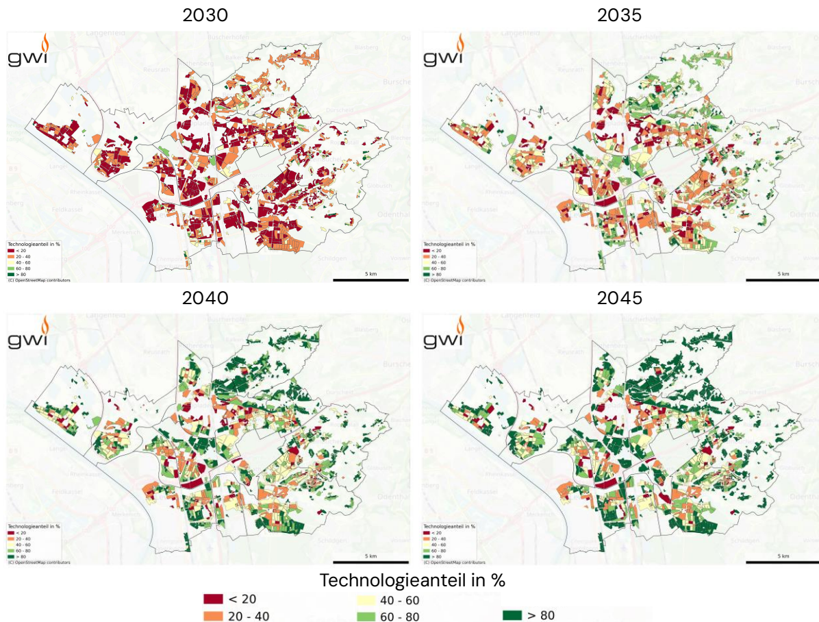
Abbildung 68: Wärmepumpen im maßgeblichen Zielszenario als Technologieanteil Wärmepumpe. Baublöcke mit ausschließlich industrieller Nutzung wurden nicht berücksichtigt (Quelle: ALKIS , LANUK-BB )
