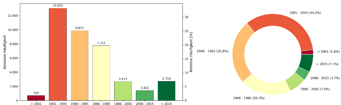
Abbildung 17: Durchschnittliches Gebäudealter im Baublock sowie statistische Verteilung auf Gebäudeebene (Quellen: ALKIS , LANUK-BB , LANUK-RBM )
