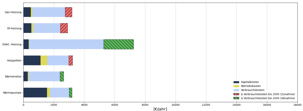
Abbildung 89: Mehrfamilienhaus saniert. Wohnfläche = 300m 2 , Wärmeleistung = 8,8 kW, Wärmebedarf = 15 MWh/a (eigene Darstellung)
