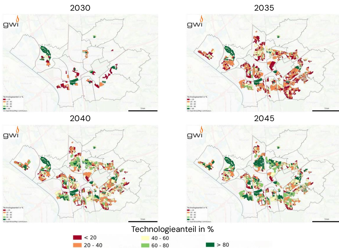
Abbildung 69: Wärmenetzversorgung im maßgeblichen Zielszenario als Technologieanteil Wärmenetz. Bau- blöcke mit ausschließlich industrieller Nutzung wurden nicht berücksichtigt (Quelle: ALKIS , LANUK-BB )
