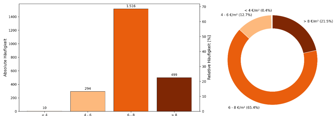
Abbildung 4: Durchschnittliche Nettokaltmiete im Stadtgebiet (Quelle: Zensus )
