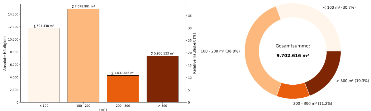
Abbildung 14: Median der beheizten Nutzfläche im Baublock sowie statistische Verteilung auf Gebäudeebene (Quellen: ALKIS , LANUK-BB , LANUK-RBM )
