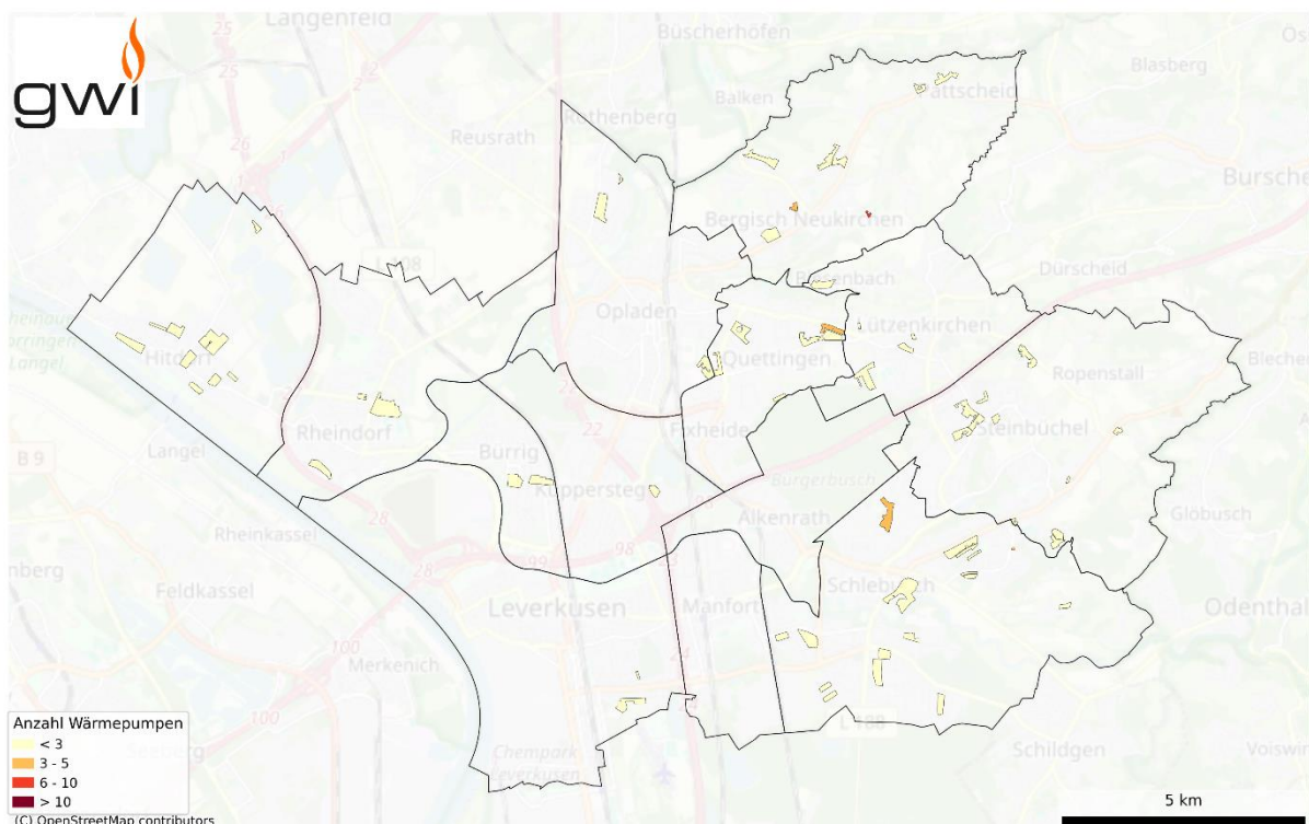
Abbildung 32: Anzahl der Gebäude mit Wärmepumpen als Heiztechnologie (Quellen: ALKIS , LANUK-BB , RNG-NSH/WP )
