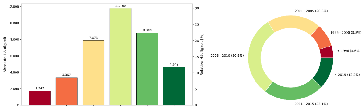
Abbildung 35: Durchschnittliches Installationsjahr des Heizsystems im Baublock sowie statistische Verteilung der Installationsjahre auf Gebäudeebene (Quellen: ALKIS , LANUK-BB , KD )
