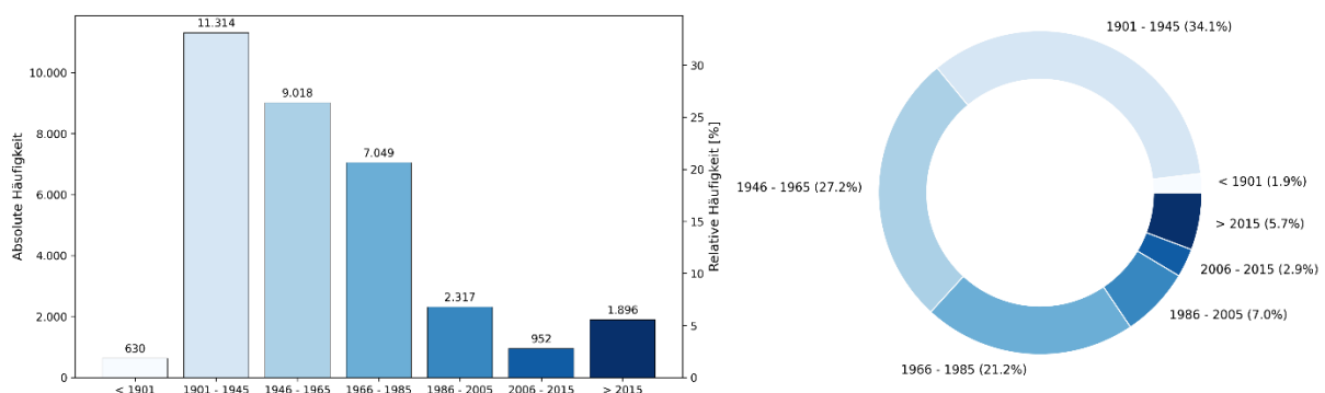
Abbildung 12: Geografische Verteilung des Wohnsektors sowie Verteilung der Baualtersklassen (Quellen: ALKIS , LANUK-BB , LANUK-RBM )
