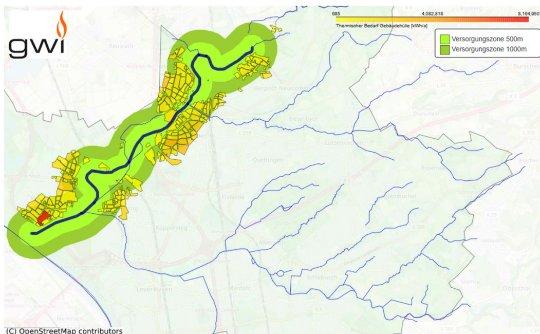
Abbildung 60: Teilausschnitt der Wupper mit Versorgungszonen (500 m Radius, 1000 m Radius) sowie Darstellung der Wärmebedarfe der Baublöcke innerhalb der Versorgungszonen (Quellen: ALKIS , LANUK-BB , RNG-RLM , RNG-EFH/MFH , AKG )
