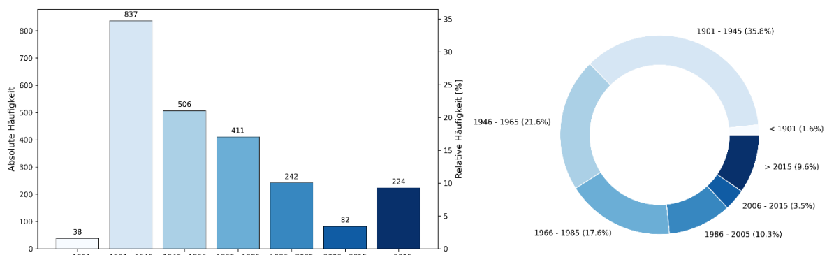
Abbildung 8: Geografische Verteilung des GHD-Sektors sowie Verteilung der Baualtersklassen (Quellen: LA-NUK-BB , LANUK-RBM , ALKIS )
