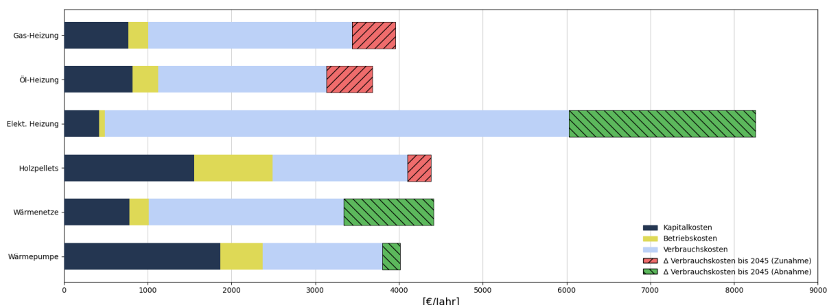
Abbildung 86: Einfamilienhaus unsaniert. Wohnfläche = 110m 2 , Wärmeleistung = 9,6 kW, Wärmebedarf = 17 MWh/a (eigene Darstellung)
