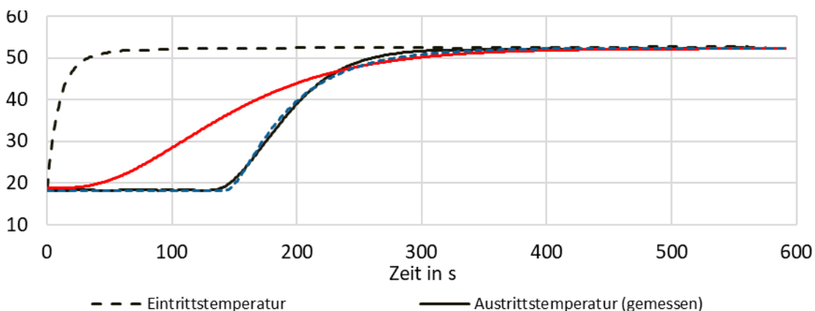
Abbildung 26: Ergebnis der Simulation eines 39 m langen Rohres mit Temperaturanstieg für ein diskretisiertes Rohrmodell und das neue Rohrmodell. Messdaten aus [Hei17]
