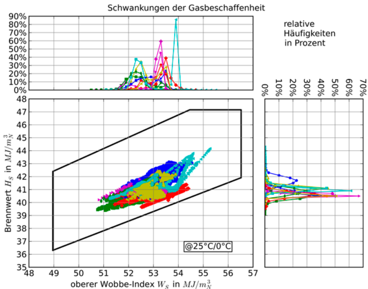
Abbildung 15: Brennwert und Wobbe-Index der untersuchten Standorte im H-Gas-Gebiet mit Häufigkeitsverteilungen des Brennwertes und des Wobbe-Index. Bezug der Häufigkeiten auf die Anzahl der Stundenmittelwerte je Standort [2]
