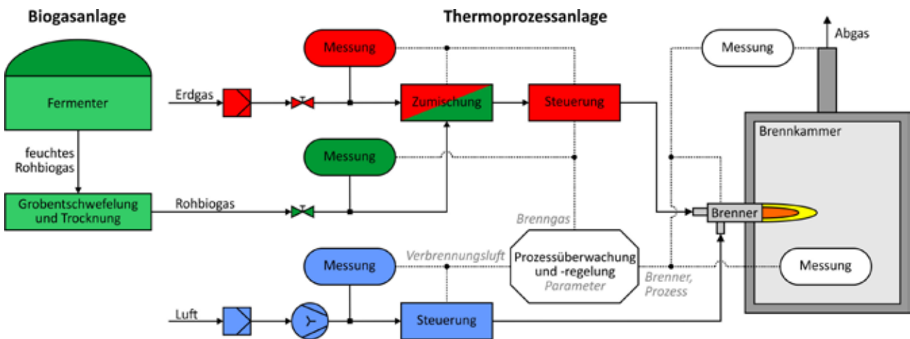
Abbildung 12: Analyse der Prozessschritte metallurgische Verfahren hinsichtlich der Eignung für die Substitution von Erdgas durch (Roh-)Biogas (Quelle: GWI)
