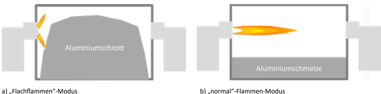
Abbildung 13: Geplante Entwicklung eines umschaltbaren regenerativen Brenners (Quelle: GWI)
