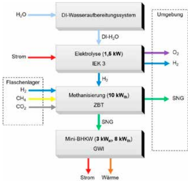
Abbildung 22: Stoffstromdiagramm der aktuell aufgebauten Anlagen
