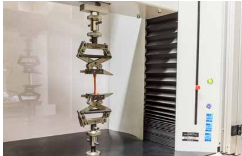
Abbildung 8: Prüfung der Mindestzugfestigkeit von Elastomerwerkstoffen
