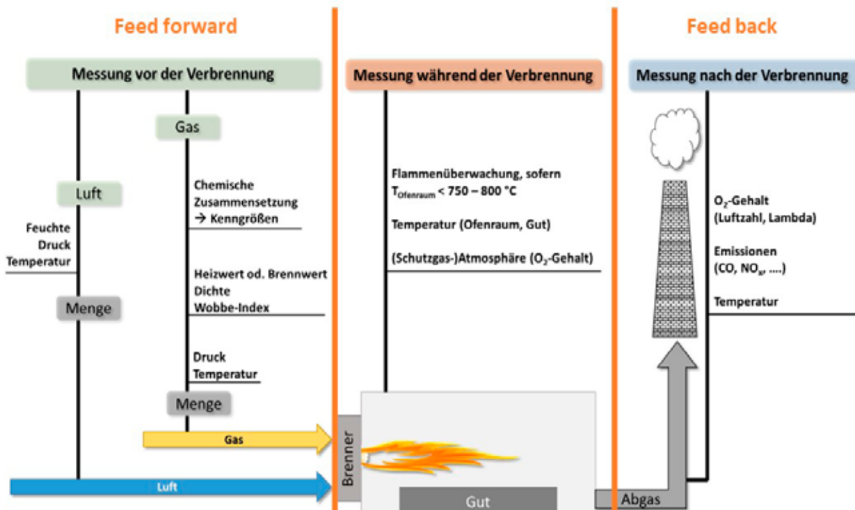
Abbildung 16: Mess- und Regelungsmöglichkeiten in einem industriellen Thermoprozess auf Basis der Ausarbeitung der SVG (Quelle: GWI/HVG)
