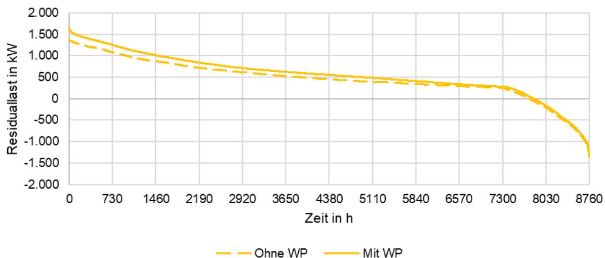
Abbildung 27: Verteilung der Residuallast über das Jahr mit und ohne Wärmepumpen-Strombezug (WP)
