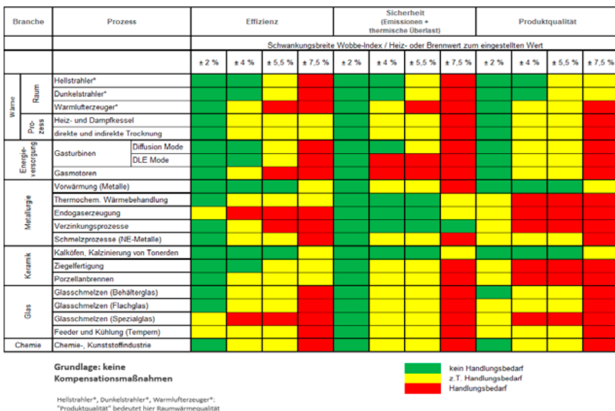
Abbildung 14: Einschätzung verschiedener Gasverwendungssysteme aus Industrie und Kraftwerkstechnik in Bezug auf schwankende Gasbeschaffenheiten [1] Seite 15 | 36
