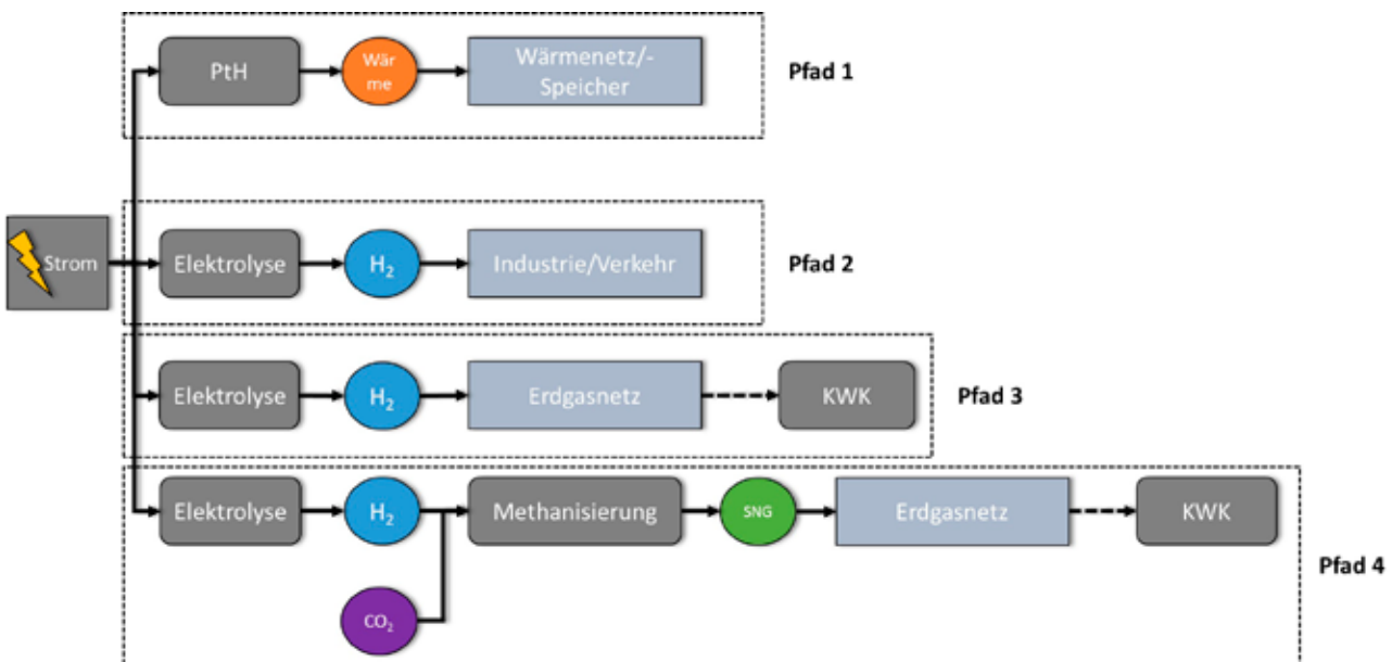
Abbildung 23: Technologiepfade der in der Demonstrationshalle implementierten Energieflexibilitätsoptionen
