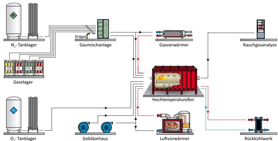
Abbildung 11: schematisches Fließbild der Hochtemperaturanlage „roter Ofen“, (Quelle: GWI)
