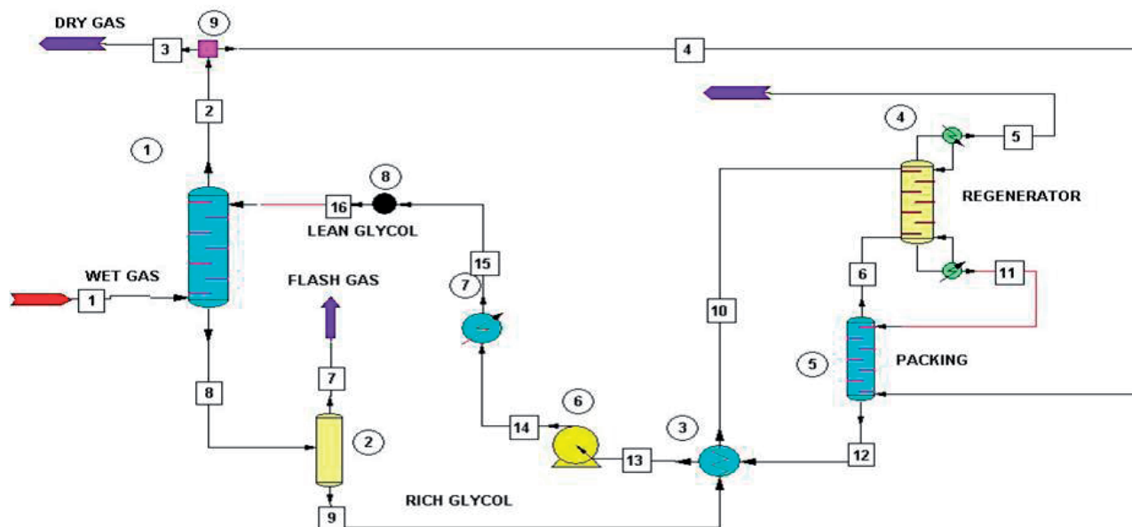
PROZESSSIMULATION EINER GASDESTILLATIONSANLAGE
