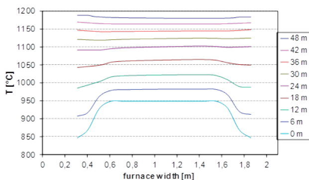
SIMULIERTE BRAMMENTEMPORATUR IN EINEM ROLLENHERDOFEN
