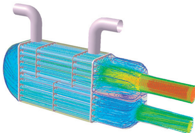
STROMLINIEN IN EINEM ABGASWÄMETAEUSCHER
