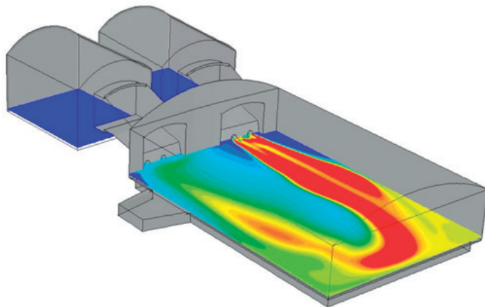
CO-VERTEILUNG IN EINER GLASSCHMELZWANNE
