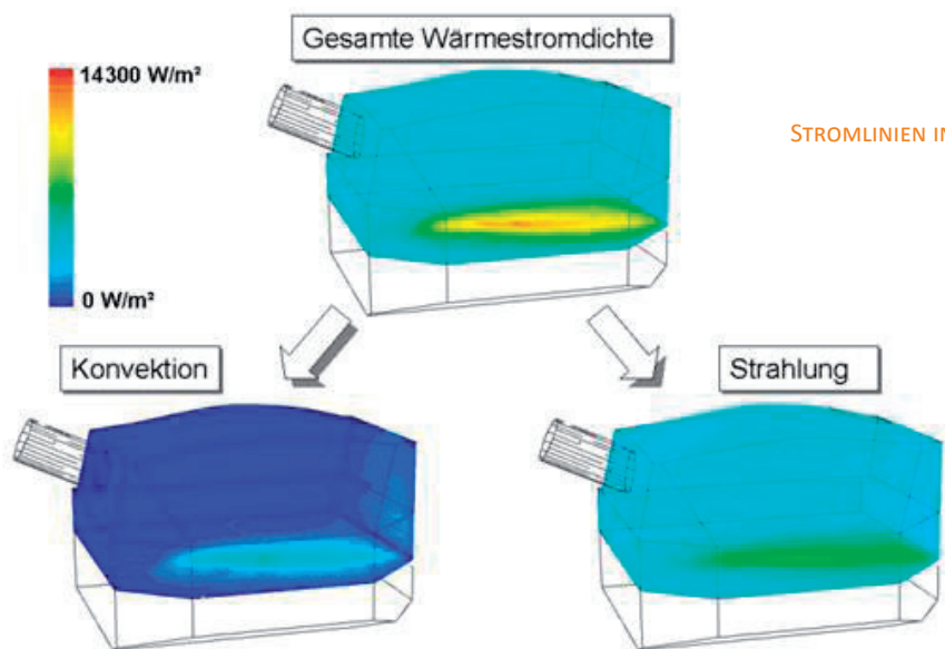
WANDWÄRMESTROMDICHTEVERTEILUNG IN EINEM ALUMINIUMSCHMELZOFEN
