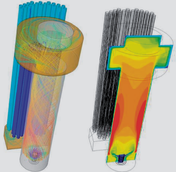
STROMLINIEN UND TEMPERATURVERTEILUNG IN EINEM INDUSTRIEKESSEL
