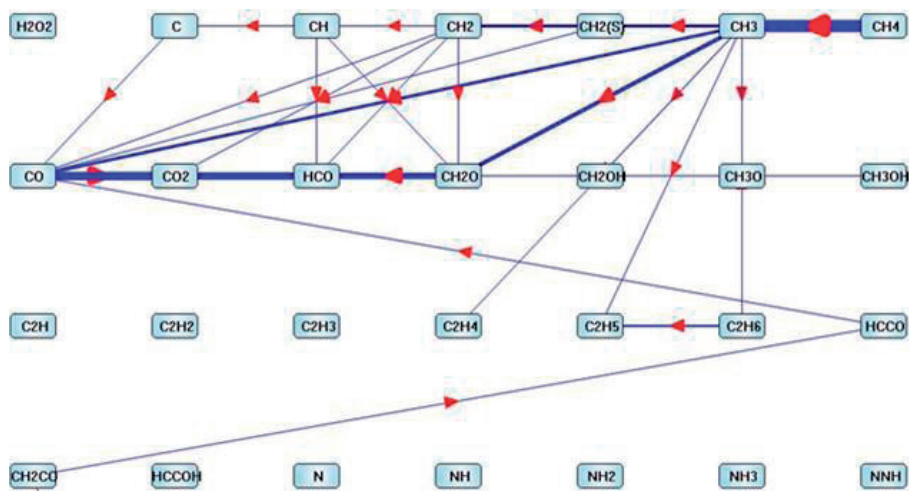
ELEMENTENFLUSSANALYSE EINER ERDGASFLAMME (AUSZUG)
